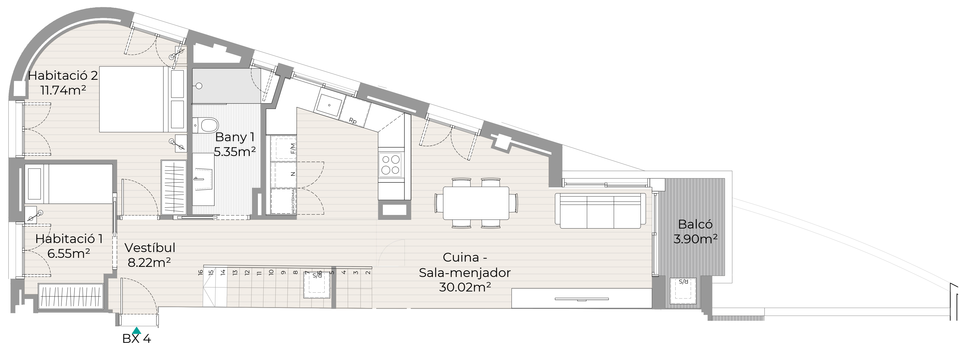
PLANTA BAIXA
