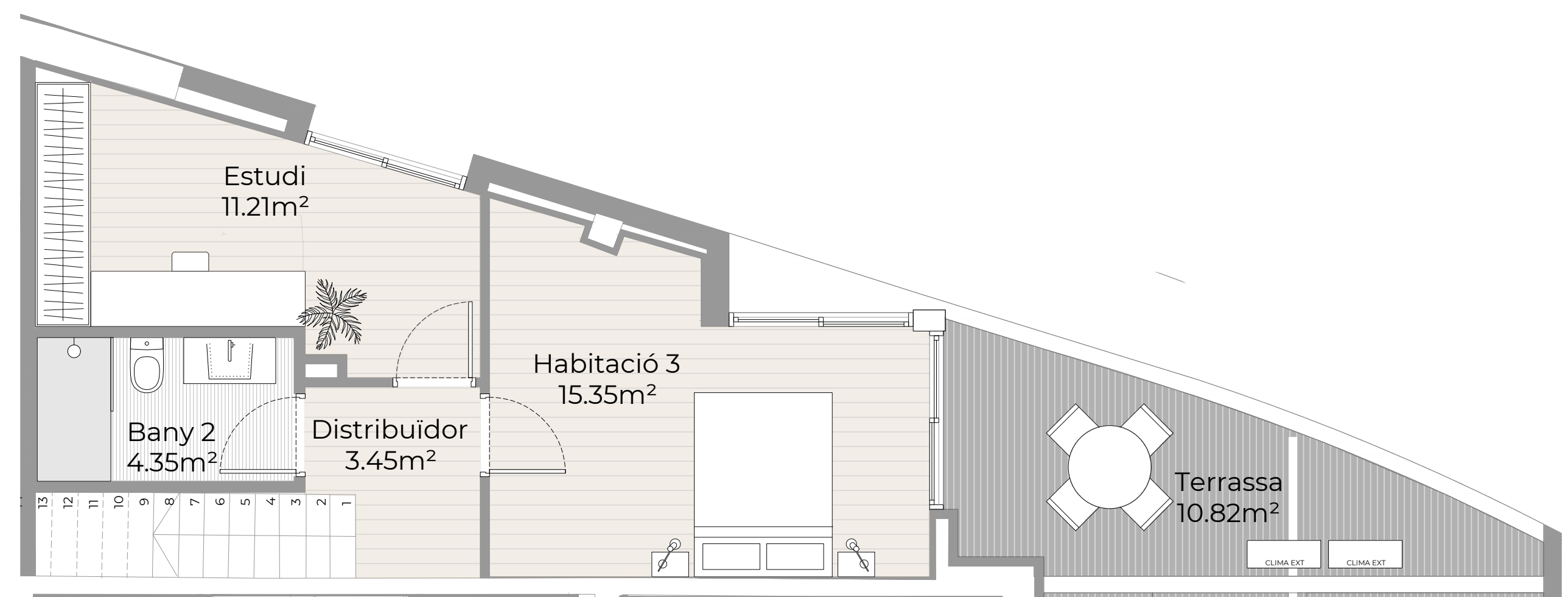
PLANTA -1
