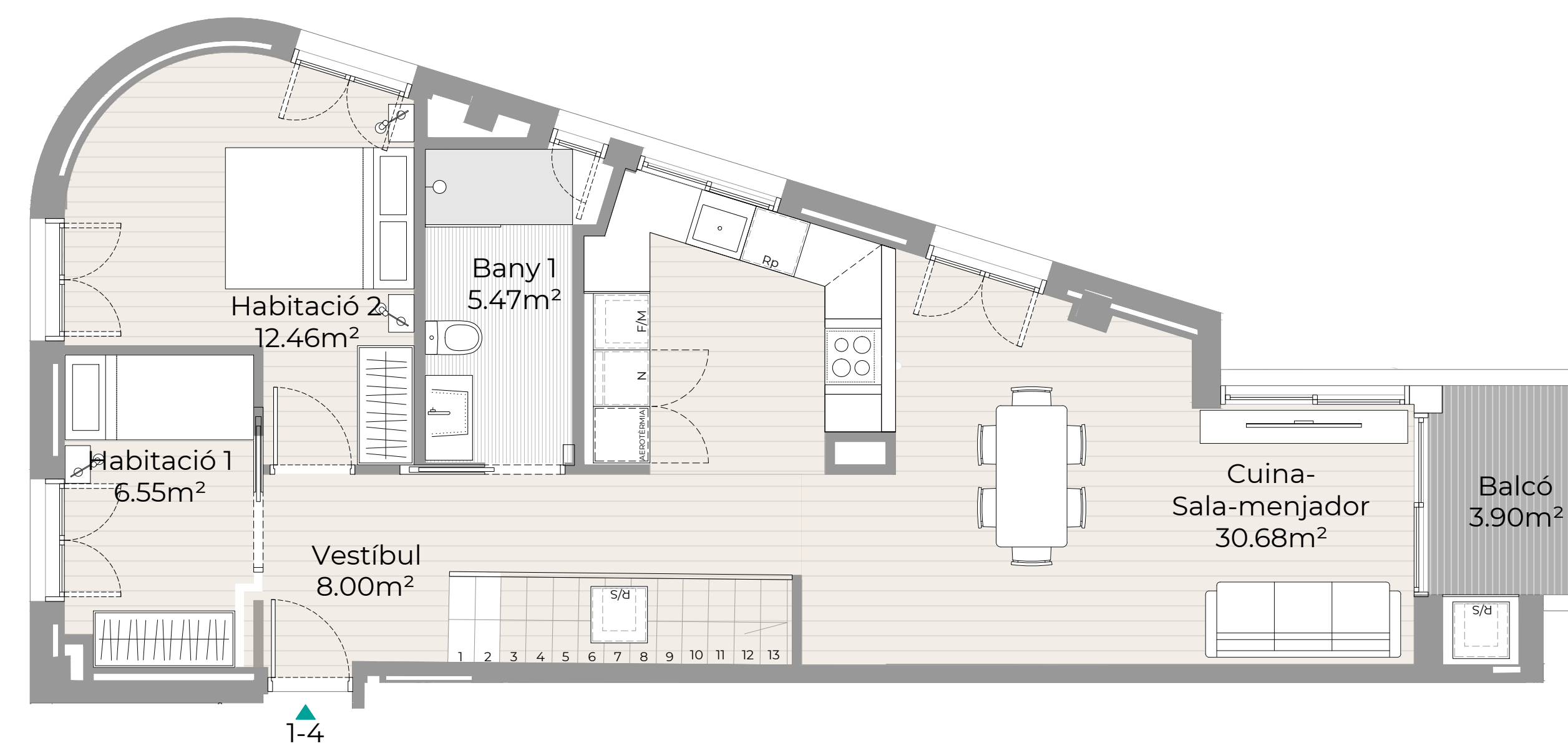
PLANTA PRIMERA
