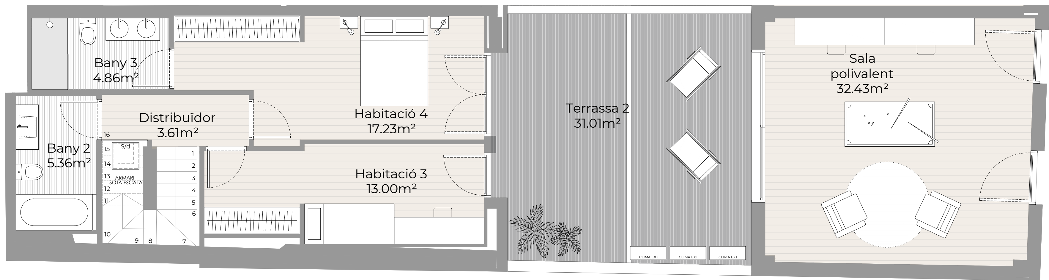
PLANTA -1
